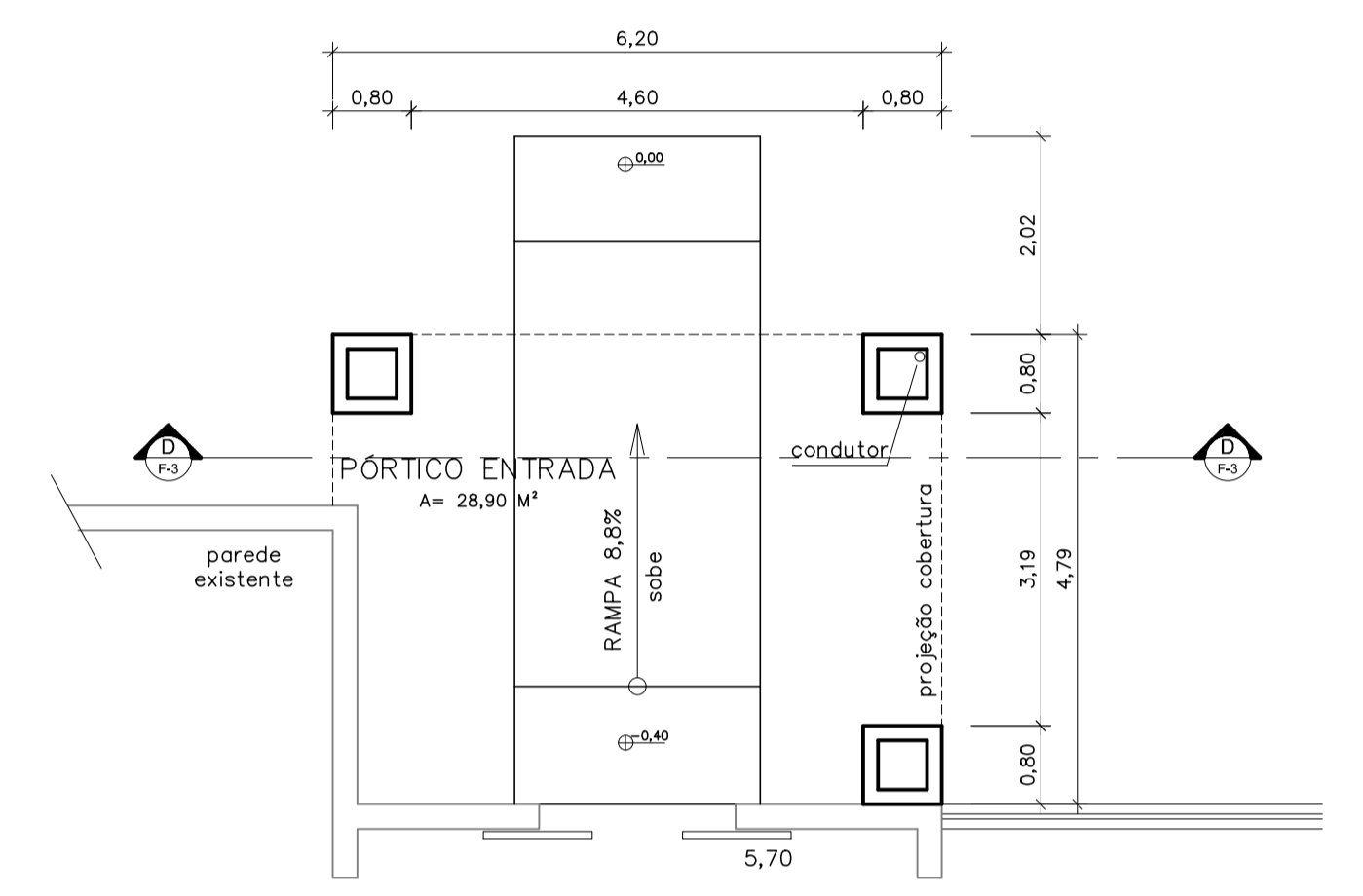
Planta Baixa - Pórtico Entrada escala 1/75
